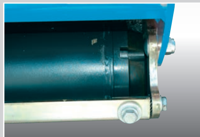
Rullo a fondelli smontabili con cuscinetti a bagno di grasso e con raschifango Roller with life-greased removable ends and mud scraper Rodillo de componentes desmontables con engrase de por vida y limpia rodillo
