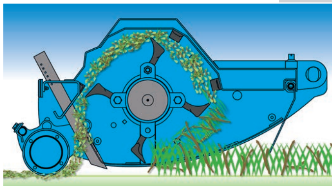
BV / BVR serie 100 – Posizione arretrata del rullo con raschiafango e denti di raccolta BV / BVR serie 100 – Backward position of the roller with mud scraper and collection rakes BV / BVR serie 100 – Posición trasera del rodillo con limpia rodillo y dientes de recogida
