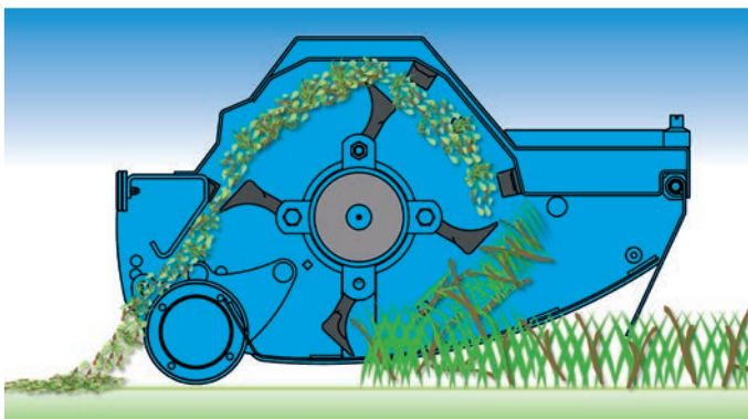
BV / BVR serie 100 – Posizione avanzata del rullo BV / BVR serie 100 – Forward position of the roller BV / BVR serie 100 – Posición delantera del rodillo
