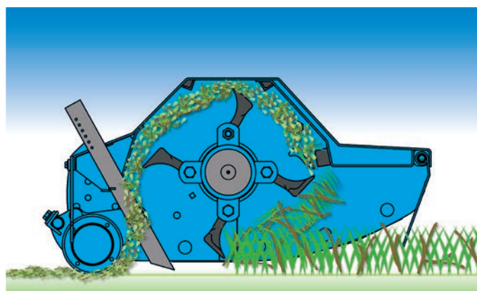
BV serie 10 – Posizione arretrata del rullo con raschifango e denti di raccolta BV series 10 – Backward position of the roller with mud scraper and collection rakes BV serie 10 – Posición trasera del rodillo con limpia rodillo y dientes de recogida
