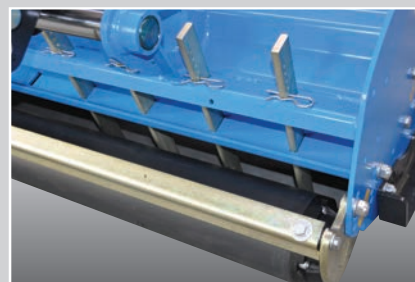
Denti di raccolta regolabili Adjustable collection rakes Dientes de recogida regulables
