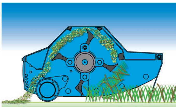
BV serie 10 – Posizione avanzata del rullo BV series 10 – Forward position of the roller BV serie 10 – Posición delantera del rodillo
