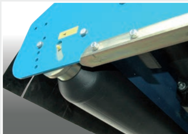
Rullo Ø 140 mm a fondelli fissi regolabile in 5 posizioni Roller: Ø 140 mm with fixed ends adjustable in 5 positions Rodillo: Ø 140 mm con extremos fijos en 5 posiciones
