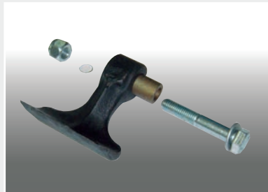
Mazza brevettata su boccia temprata e perno trattato Patented hammer on heat treated bushing and hardened axle Martillo patentado sobre casquillo guía templado y perno tratado
