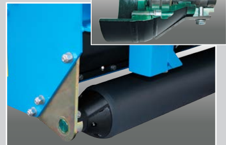
Rullo d'appoggio con fondelli smontabili, labirinti e guarnizioni su cuscinetti lubrificati a vita. Roller with removable ends, labyrinths and seals on life-greased bearings Rodillo de apoyo con componentes desmontables, labirintos y juntas en rodamientos engrasados de por vida
